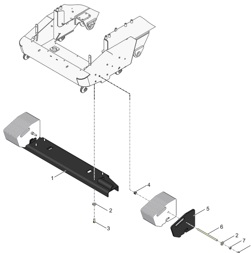
Рисунок 1 – Демонтируемые сборочные единицы и комплектующие
